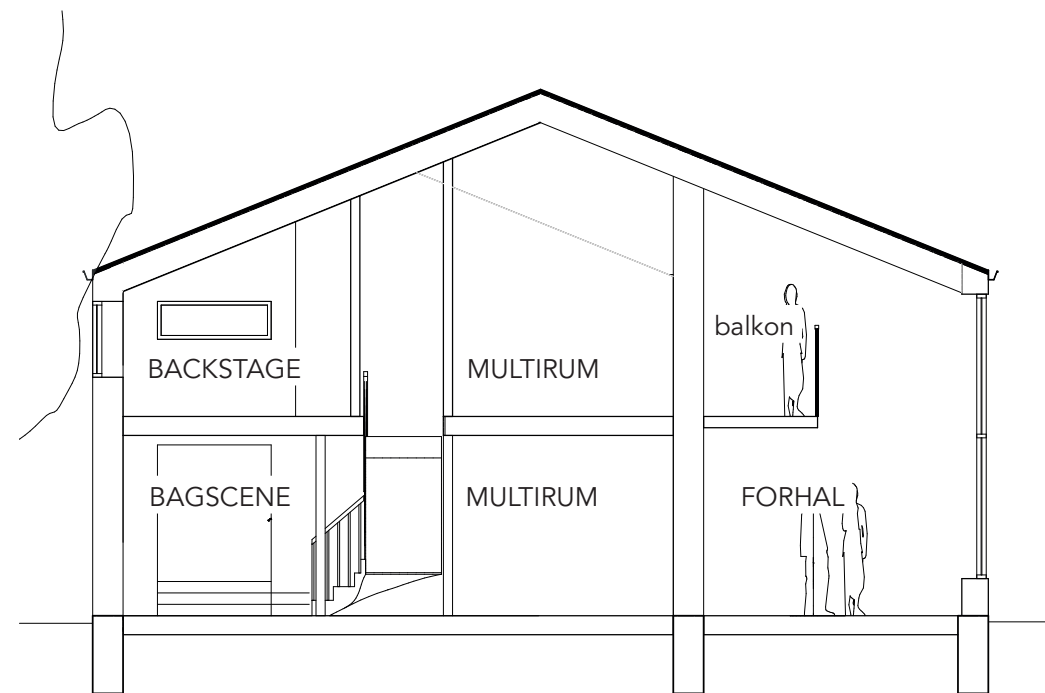
SNIT I BACKSTAGE OG MULTIRUM
