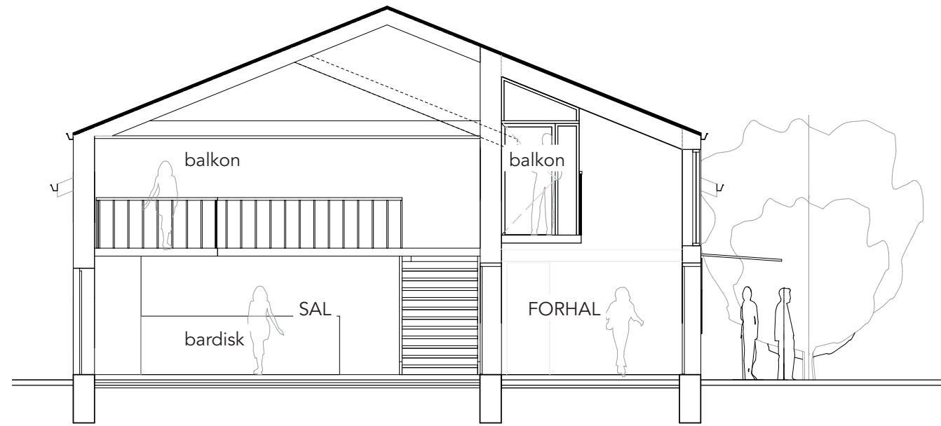
SNIT I SAL
